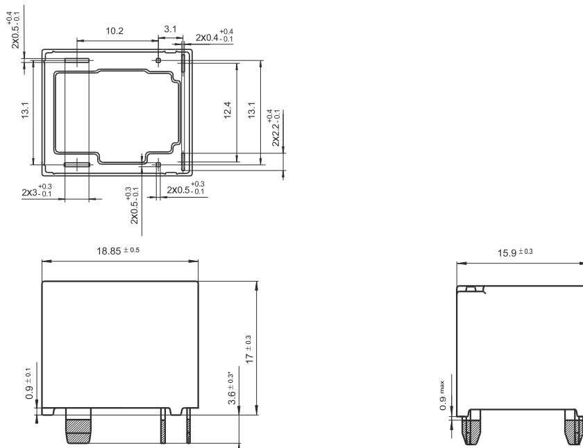
外形图
