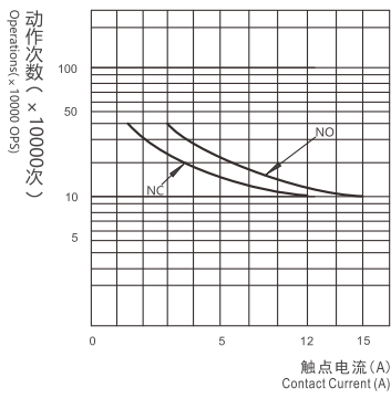
电耐久性曲线 ENDURANCE CURVE
